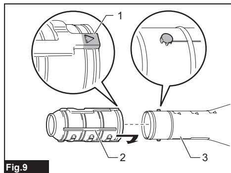
► 1. Marque triangulaire 2. Buse d'extrémité 3. Tube de souffleur
