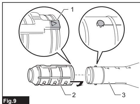
► 1. Marca de triángulo 2. Boquilla de extremo 3. Tubo de la sopladora
